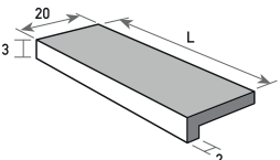
BORDE 3 EDGE 3 20xL 20x61 / 20x75 P 41 P 44
